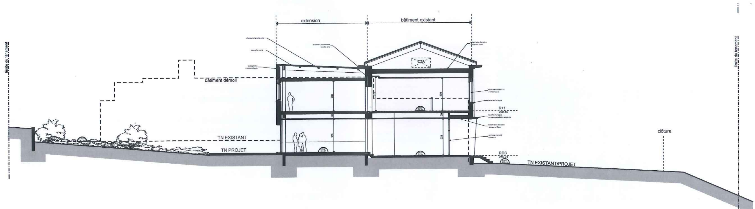
coupe 2 - sur le bâtiment A
